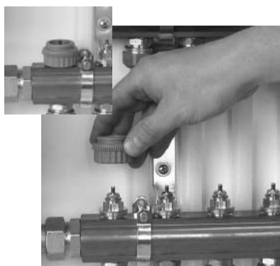
Skrue den medfølgende plastadapter på ventiltoppen
